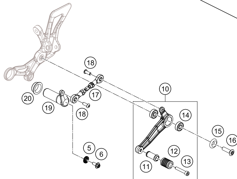
SCHALTHEBEL DUKE R SHIFT LEVER DUKE R
